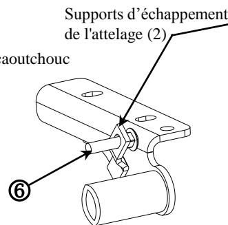
Supports d'échappement de l'attelage (2) ÉTAPE 3 Doit être installé avant de soulever l'attelage en position.
