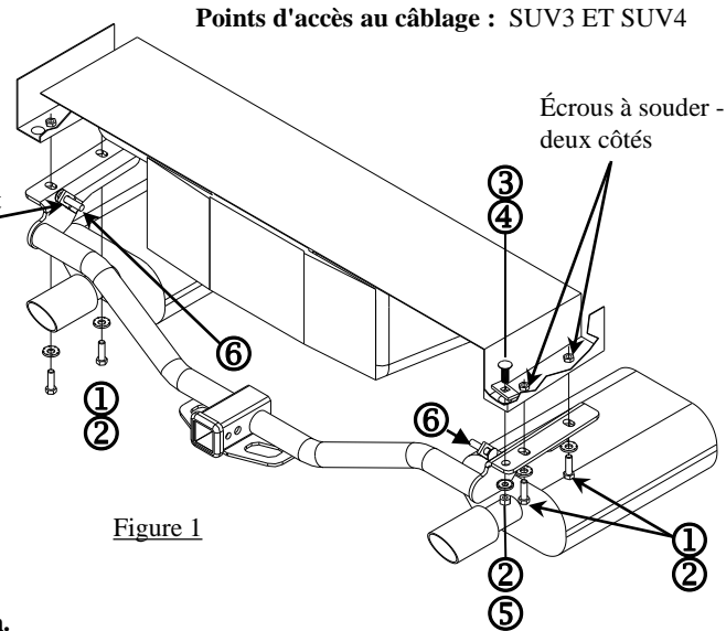
Supports d'échappement de l'attelage (2) ÉTAPE 3 Doit être installé avant de soulever l'attelage en position.
