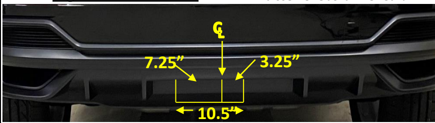
Figure 3 - Vue arrière
