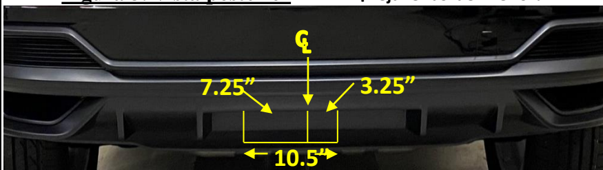
Figura 3. Vista posterior
